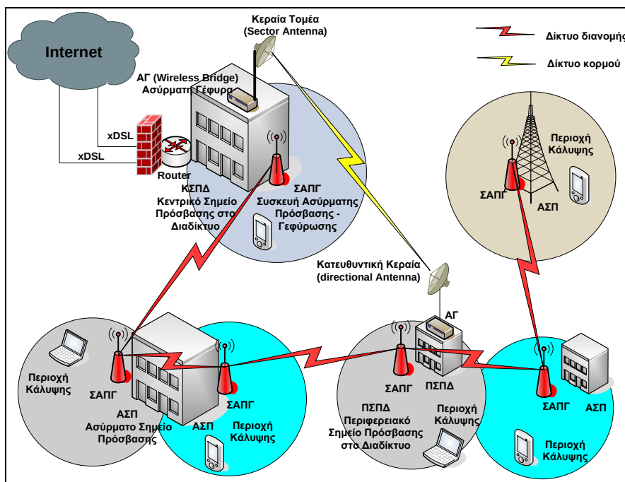
Ενδεικτική διάταξη επιμέρους κατανεμημένου ασύρματου δικτύου
